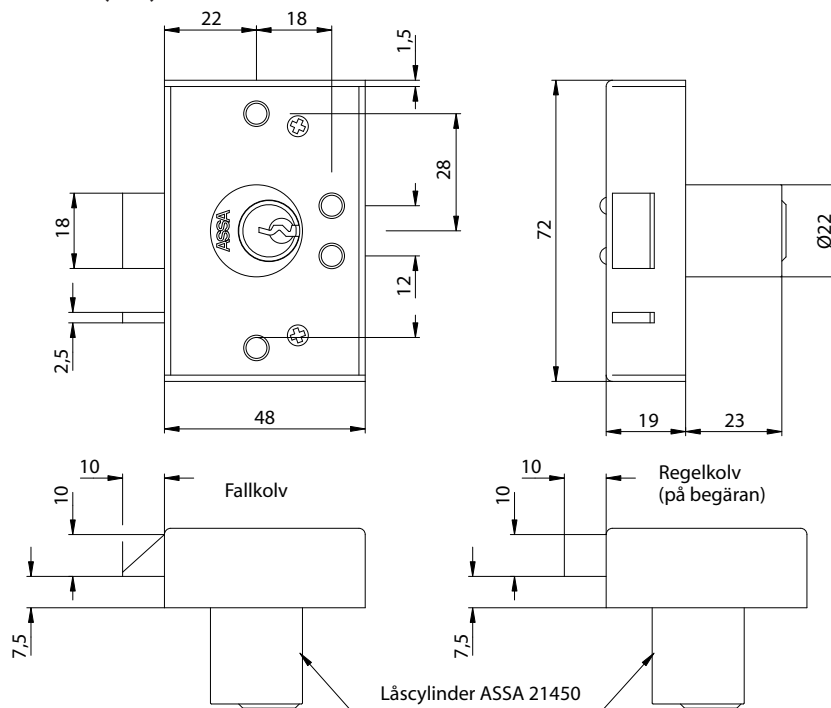
Måttskiss (mm)
