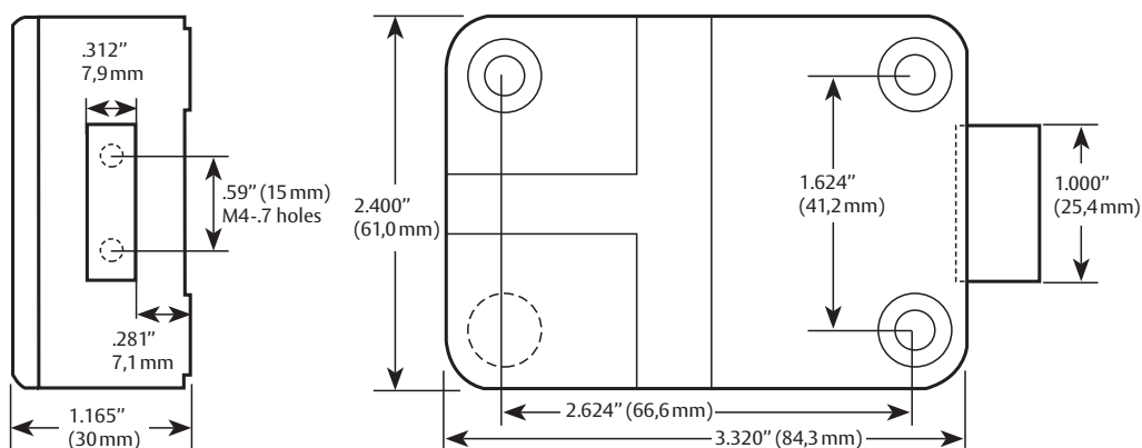
Måttskiss
