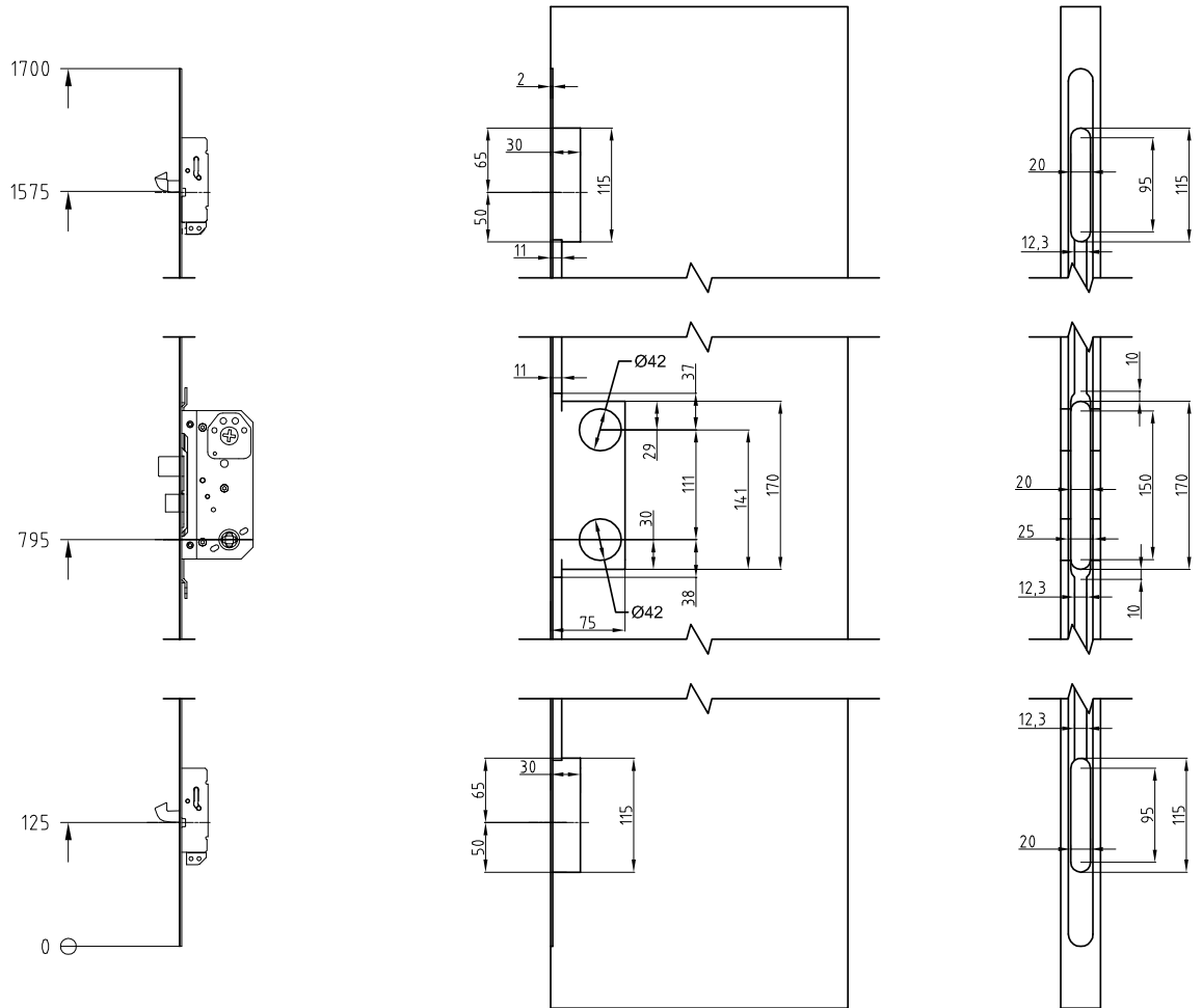
Urfärningsritning ASSA Modul 8765 MPL.*
