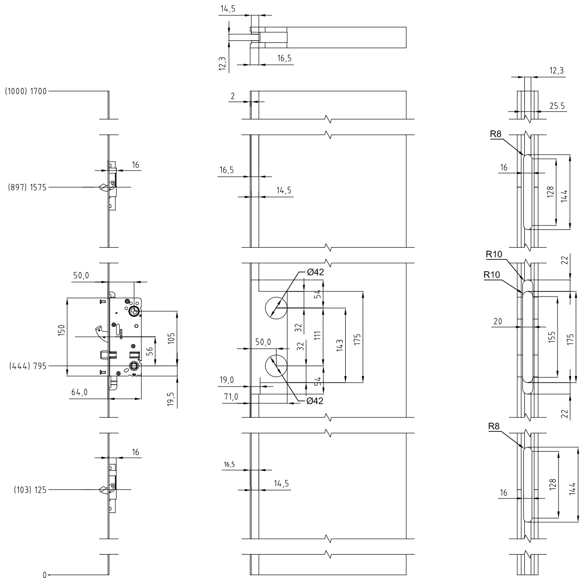
Mått ritning ASSA Connect 310 MPL*
