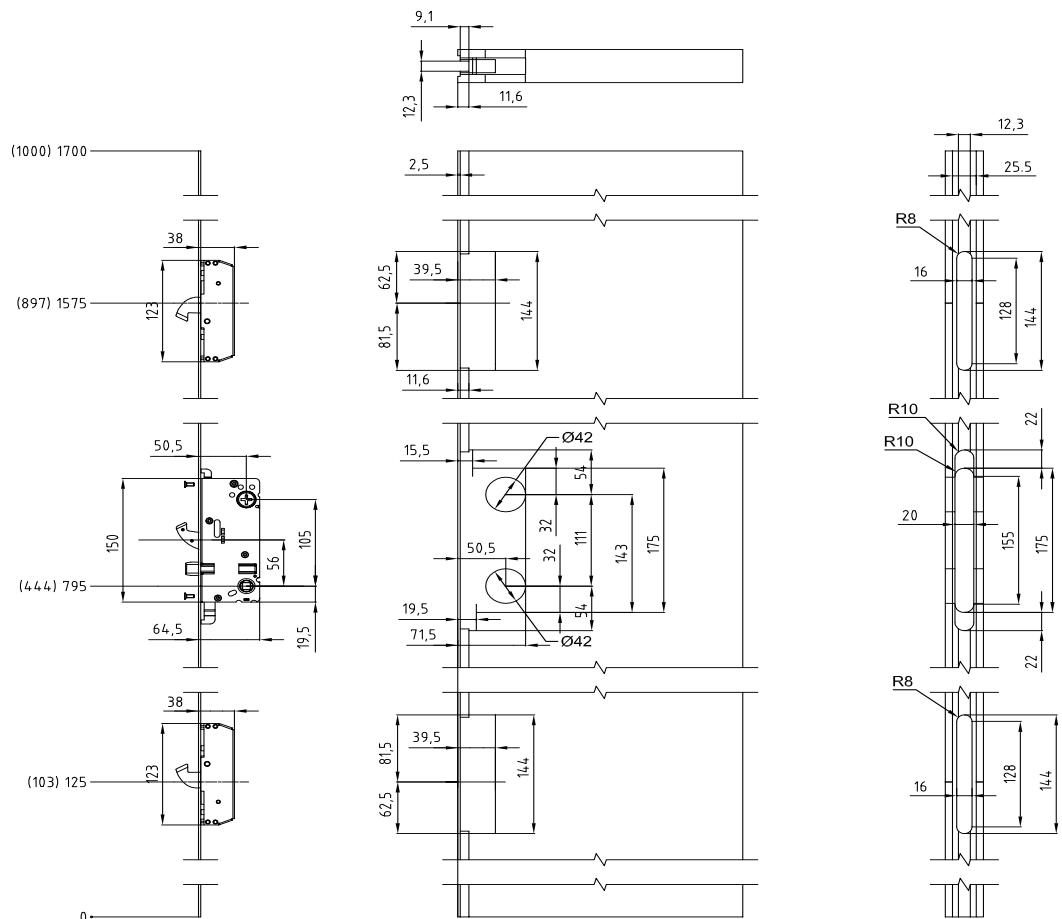
Mått ritning ASSA Connect 410 MPL*
